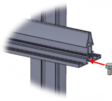
2- Glisser une vis H M6x10
